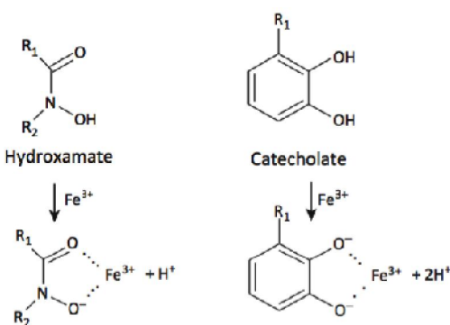
شکل 3- روش به دام انداختن آهن سه ظرفیتی توسط برخی سیدروفورها
